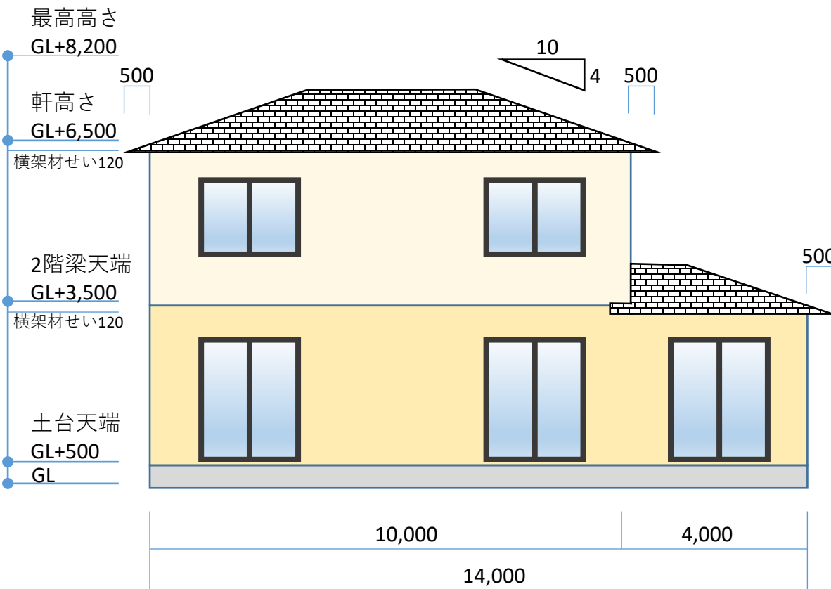
■ 南側立面図
