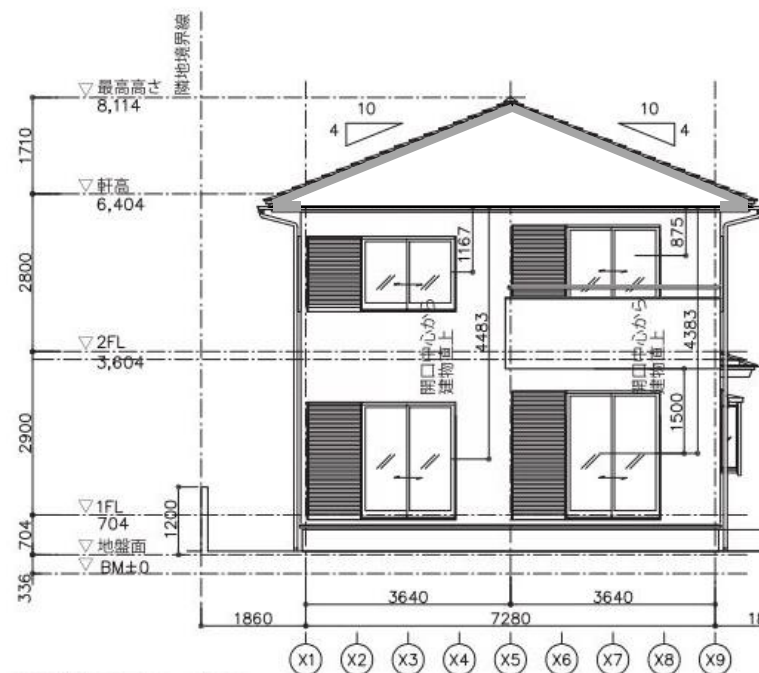
■南側立面図
