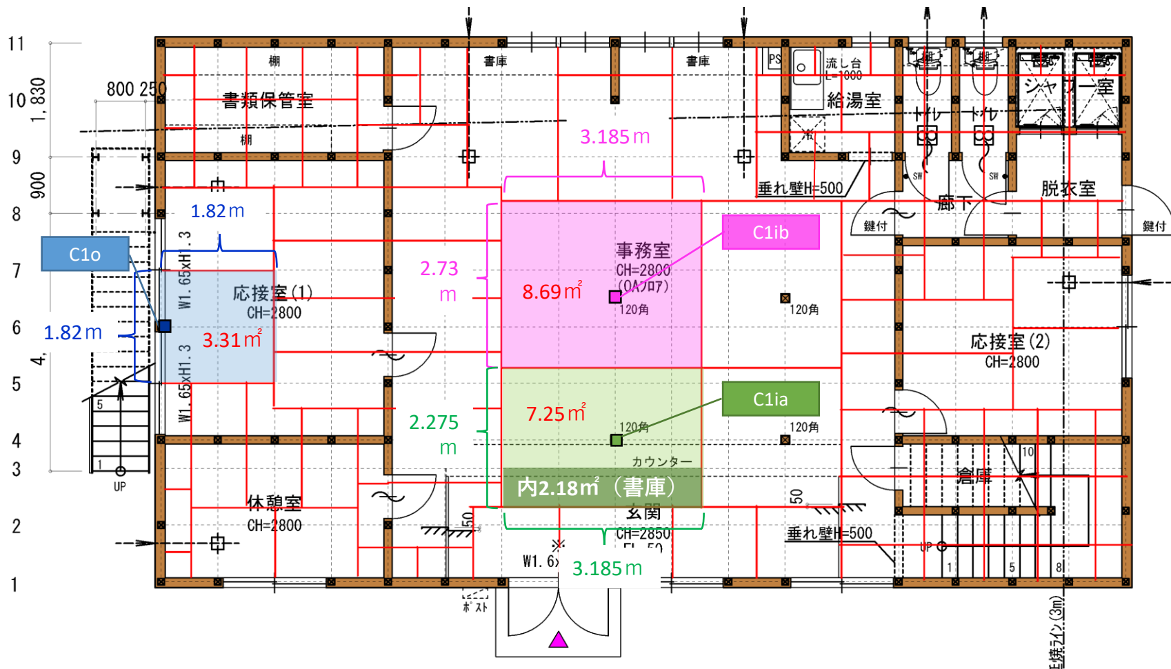
1階平面図
