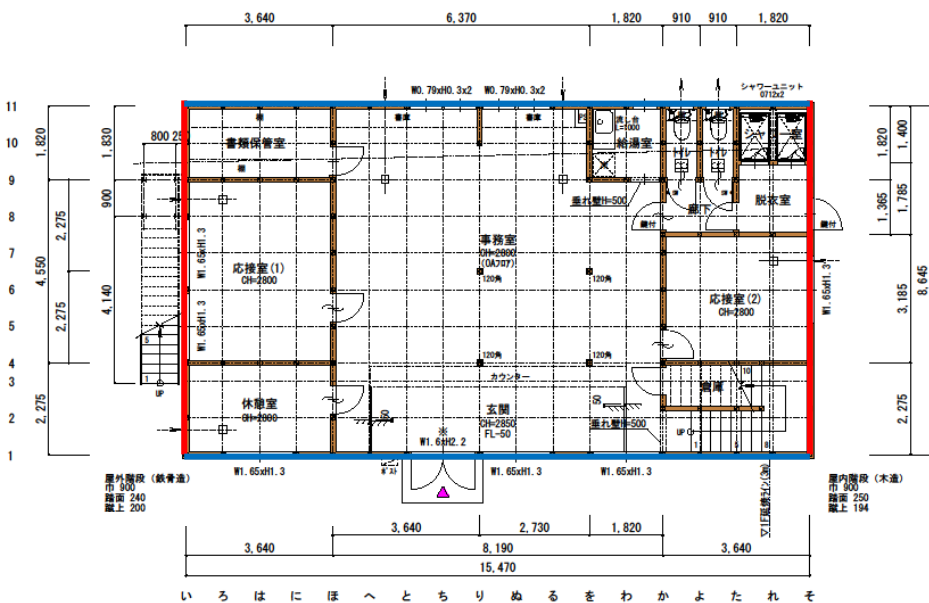
■ 1階平面図
