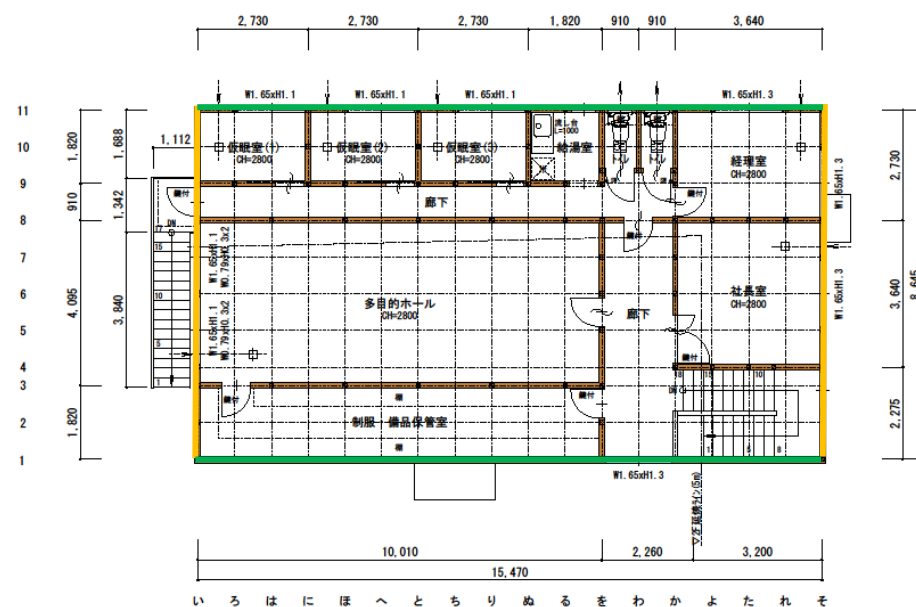
■ 2階平面図
