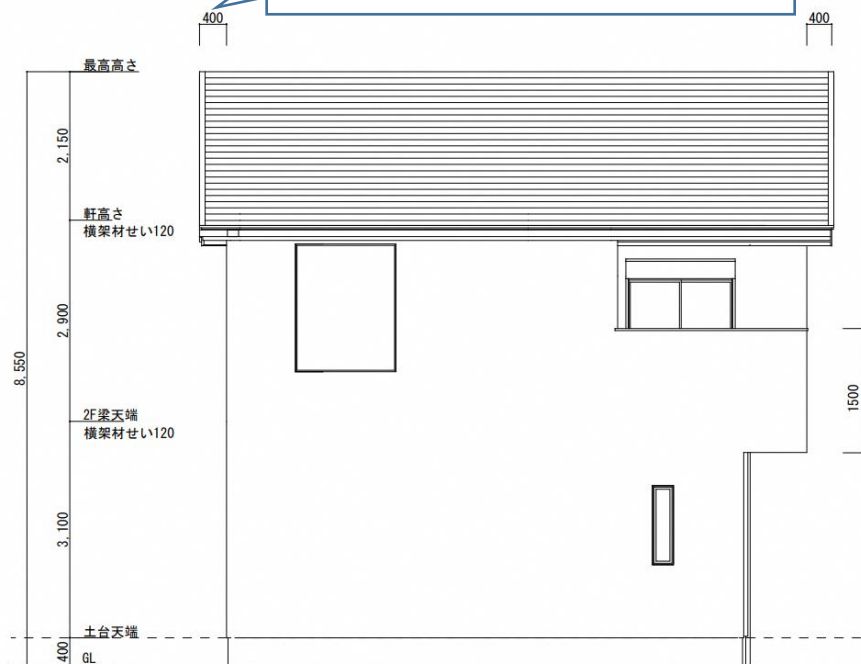
南面立面図
